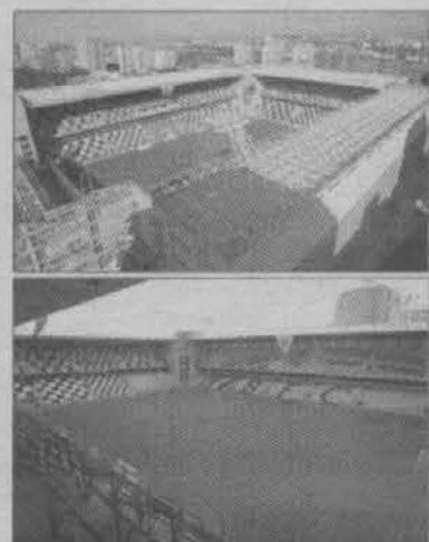
«Эштадью ду Бесса Секулу XXI» Место расположения: Порту. Владелец: футбольный клуб «Боавишта». Вместимость: 28,263 зрителя. Архитектор: «Группа 3». Дата открытия: 30 декабря 2003 года. Стоимость строительства: 45.164.726 евро.
